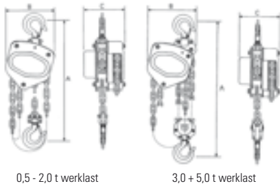
0,5 - 2,0 t werklust
