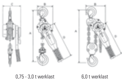
0,75 - 3,0 t werklust
